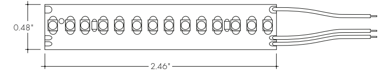
LLDW68-HO
